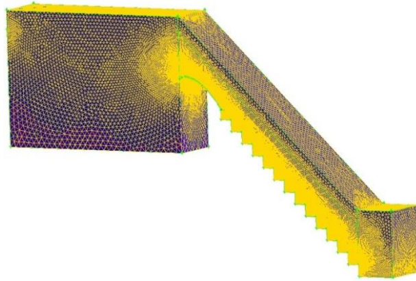
شکل ۱- شبکه بندی مدل بوسیله ی نرم افزار GAMBIT
