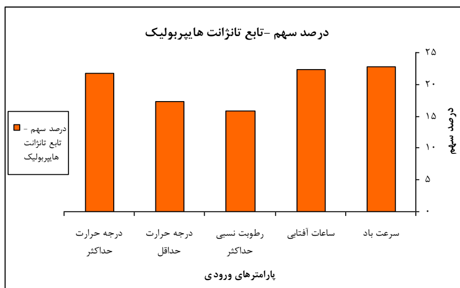
شکل ۴- درصد اثرگذاری پارامترهای ورودی در ساختار نهایی بدون رطوبت نسبی حداقل
